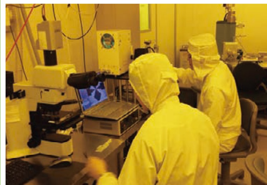
クリーンルーム（イエロールーム）内での半導体微細加工プロセスの様子
